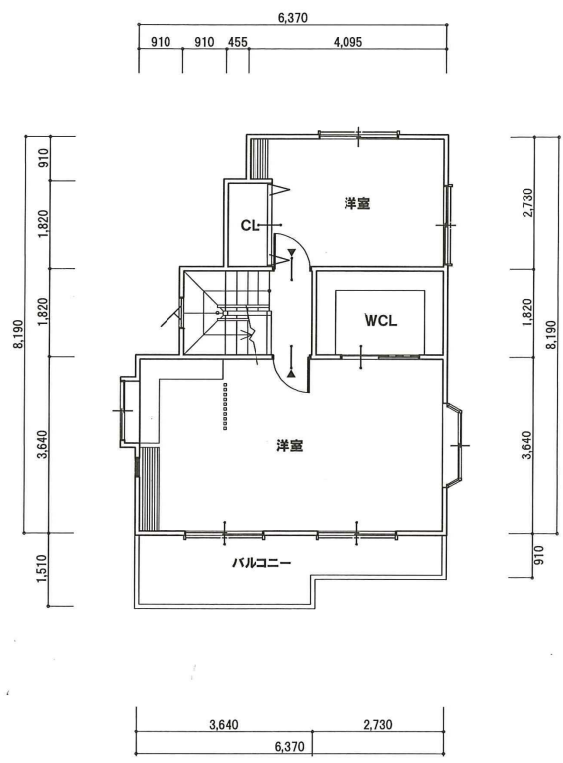
3階 平面図 S:1/100
